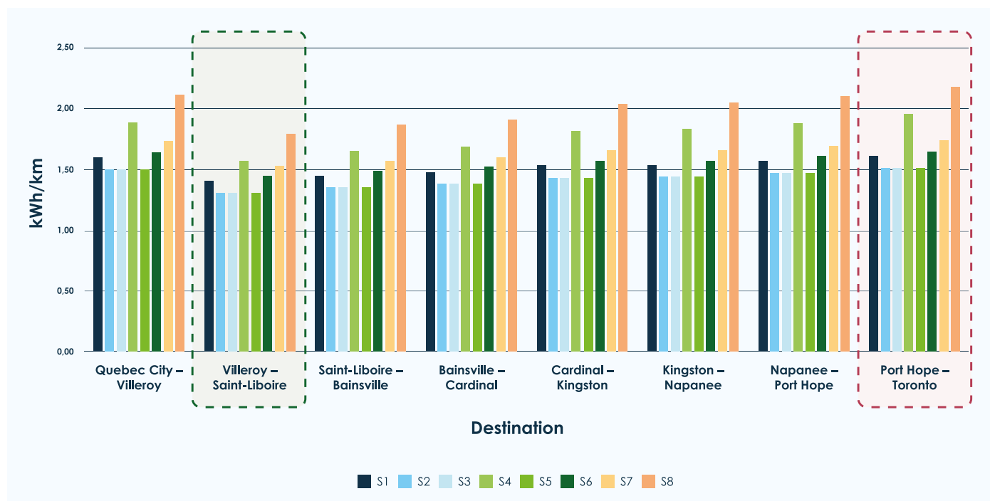
Figure 4-5 : Consommation énergétique moyenne en fonction des tronçons
